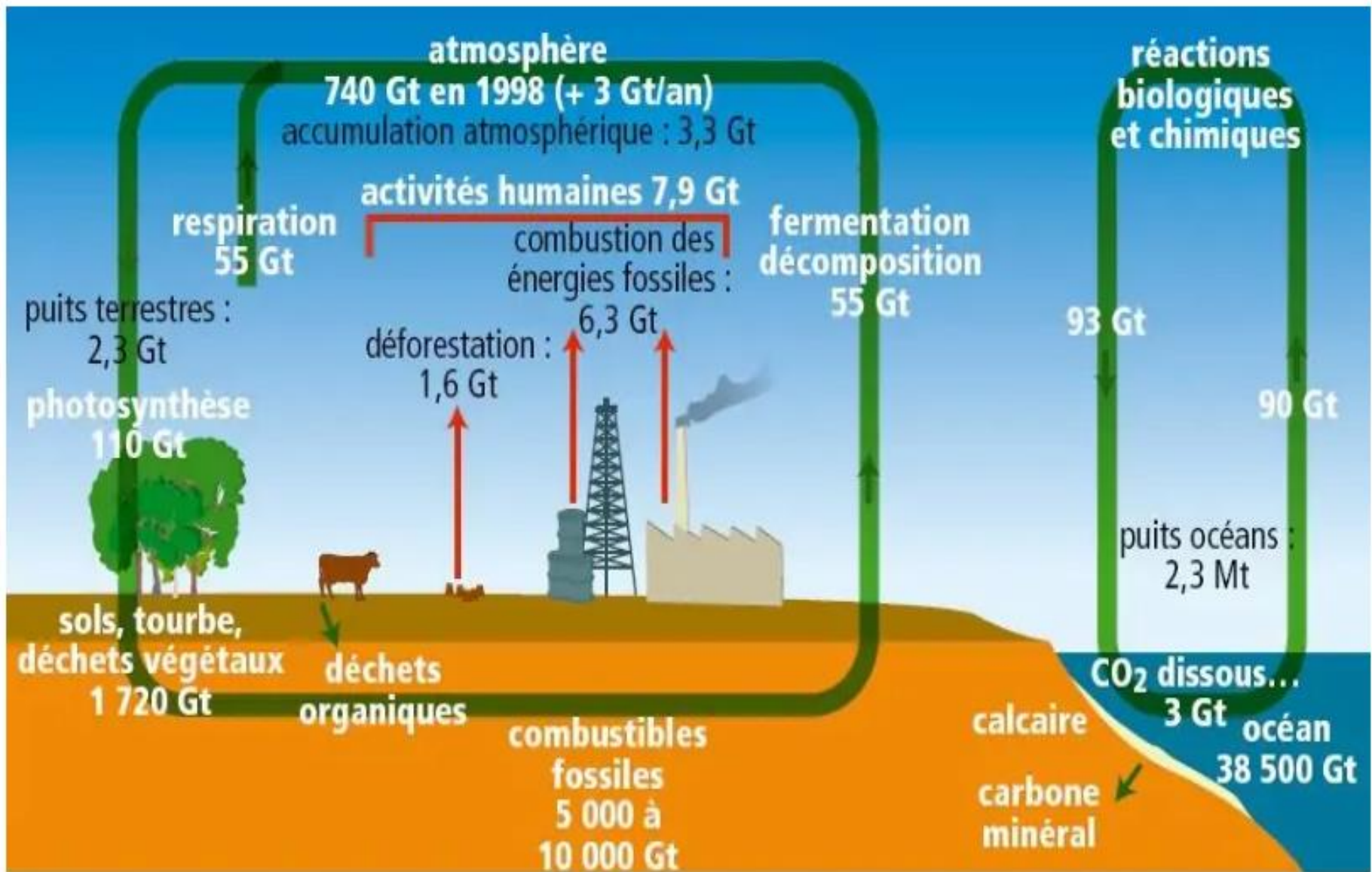
Schématisation des flux annuels planétaires de carbone
